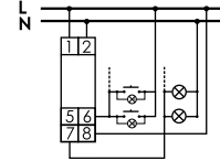
4 vezetékű bekötés
