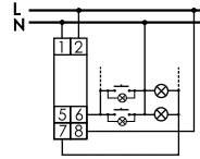
3 vezetékű bekötés
